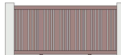
Autan C (5) Remplissage vertical Lames de 40, 80 (2 lames) et 160 mm
