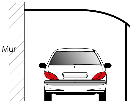
▲ Exemple A - Toit asymétrique Pose contre mur + 2 ou 3 poteaux
